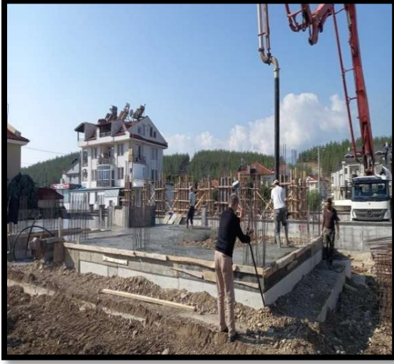
Foto-1: Subasman Kontrolünden Bir Görünüm
